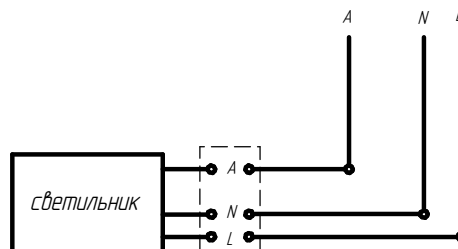
Рисунок 3 - Схема подключения светильника с БАП к сети, схема подключения светильника с микроволновым датчиком и БАП к сети.
