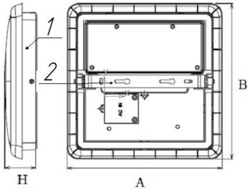
Рисунок 1: Светильники серии ДБО89; 1 - Корпус в сборе; 2 - Скоба.
