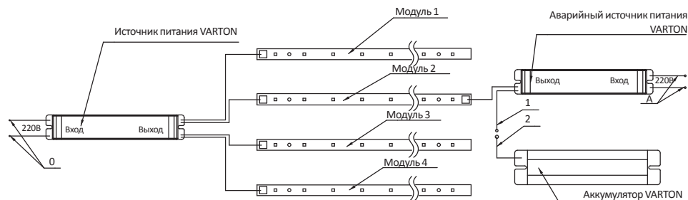
Рис. 1 Типовая схема подключения.
