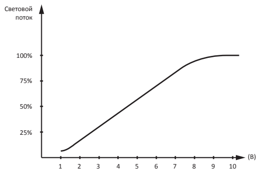
Рис. 3 . Зависимость светового потока от диммера.
