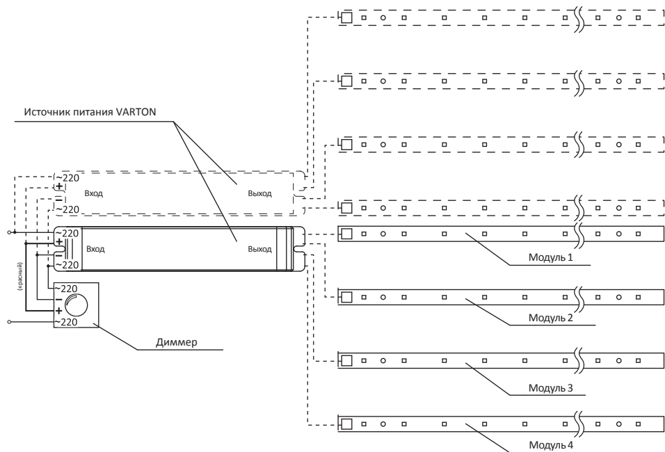
Рис. 2 . Схема подключения с диммером.
