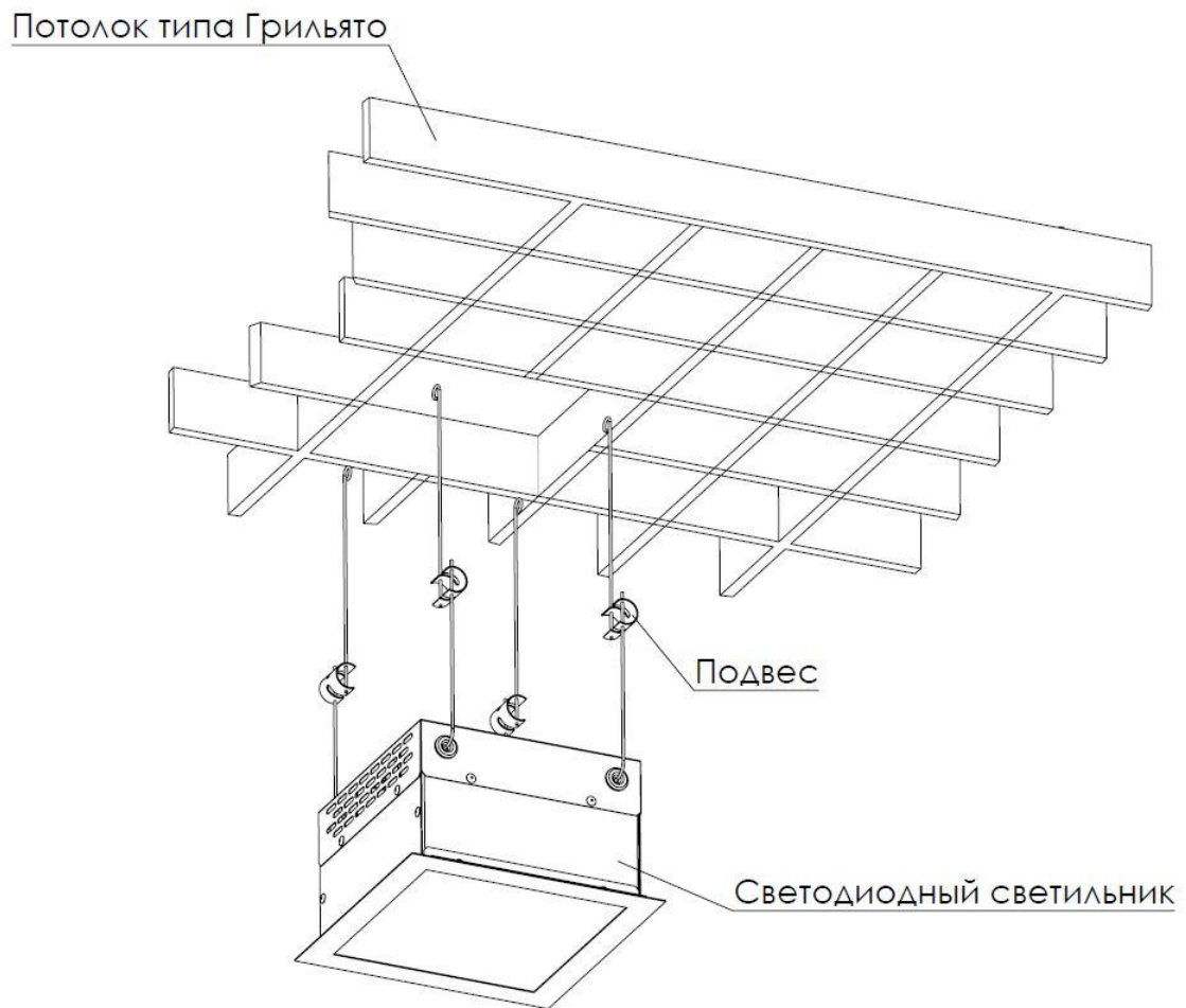
Рис.2 – Схема крепления подвесов к светильнику
