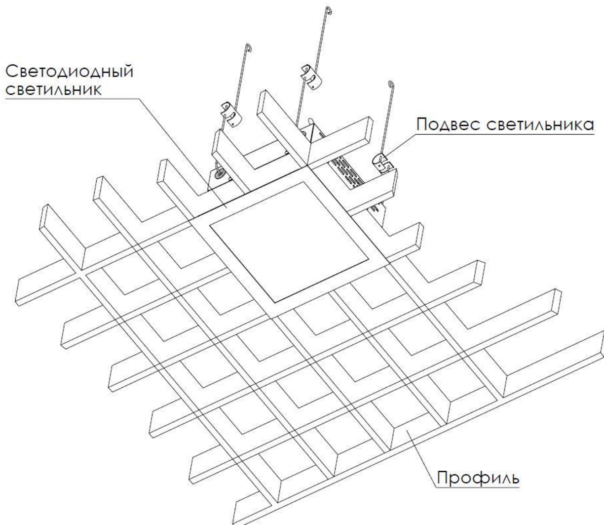
Рис.3 – Схема установки светильника серии «Грильято» в реечный потолок.
