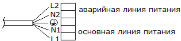
Схема подключения светильника с аварийным блоком
