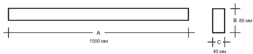
Габаритные размеры светильника
